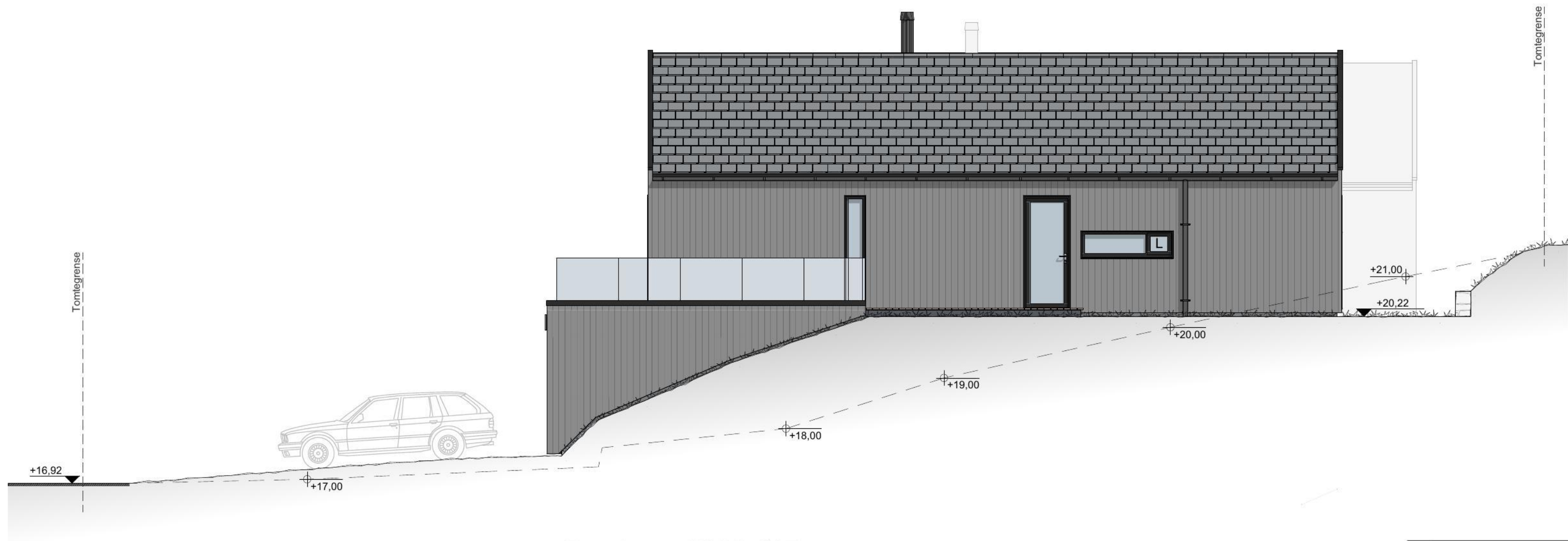
Fasade mot NORD-ØST bolig A
